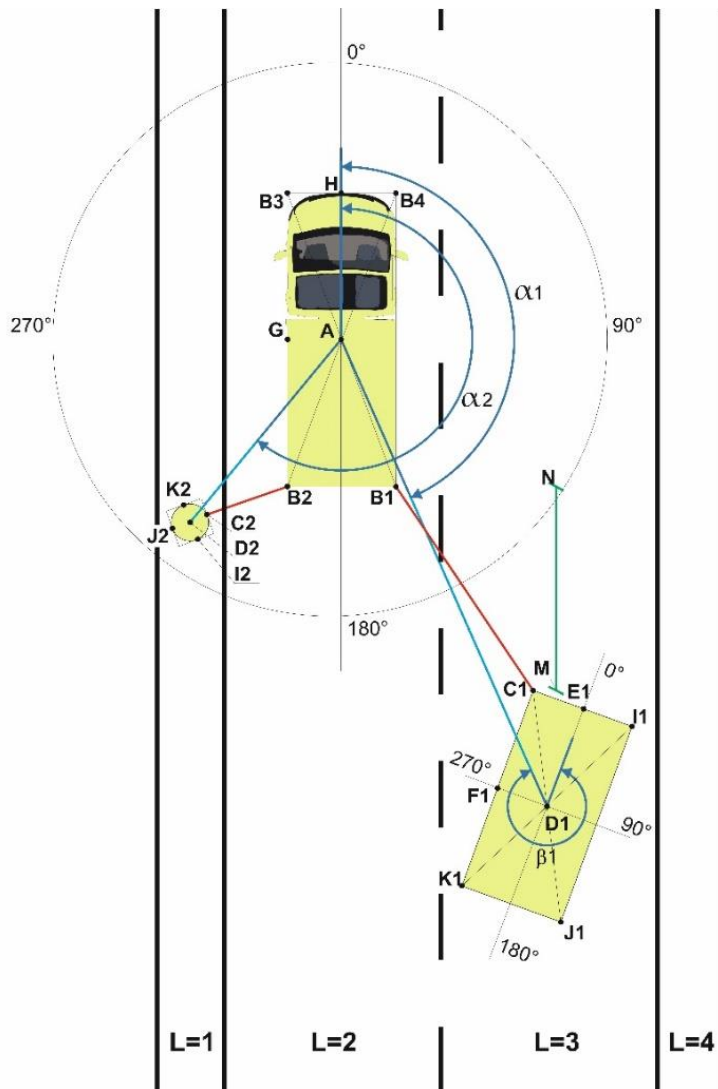
Рисунок 3.3 – Параметры БПТС и препятствий
